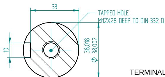
Przekrój A-A 1:1
